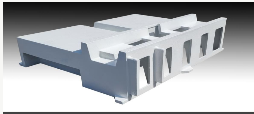
BASE Casting · FC300
